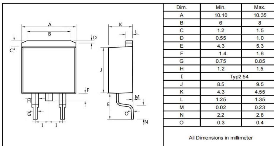
TO-263
